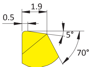
Détail A
