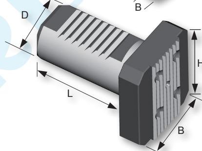
VDI-Aufnahmen
